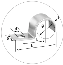
NORMAFIX® BSL ТИП 510 ДЛЯ 1 ЛИНИИ (по DIN 72571)
